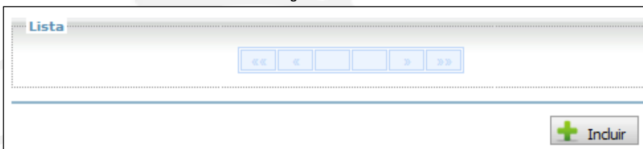
Figura 149: Lista
